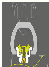
Рис. С: Регулятор отсоединен от вентиля Коннектор YOKE закрыт
