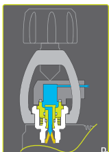
Рис. D: Регулятор подключен к вентилю Коннектор YOKE открыт
