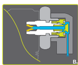
Рис. В: Регулятор подключен к вентилю Коннектор DIN открыт
