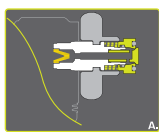
Рис. А: Регулятор отсоединен от вентиля Коннектор DIN закрыт
