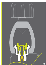
Рис. С: Регулятор отсоединен от вентиля Коннектор YOKE закрыт
